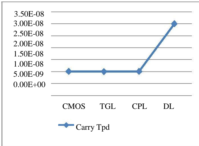
Fig. (d) Carry Propagation Delay
